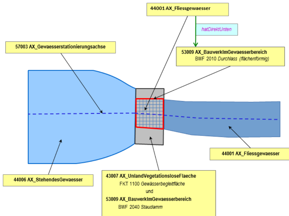
Abbildung 55: Modellierung von Wasserlauf unter Staudamm in flächenförmigem Durchlass Verläuft ein Verkehrsweg wie z. B. eine Straßenachse auf einem Staudamm oder einer Staumauer erhält dieser eine „hatDirektUnten“-Relation zum Bauwerk. Dadurch wird die Grundfläche, auf der das Bauwerk liegt, nicht geteilt.
