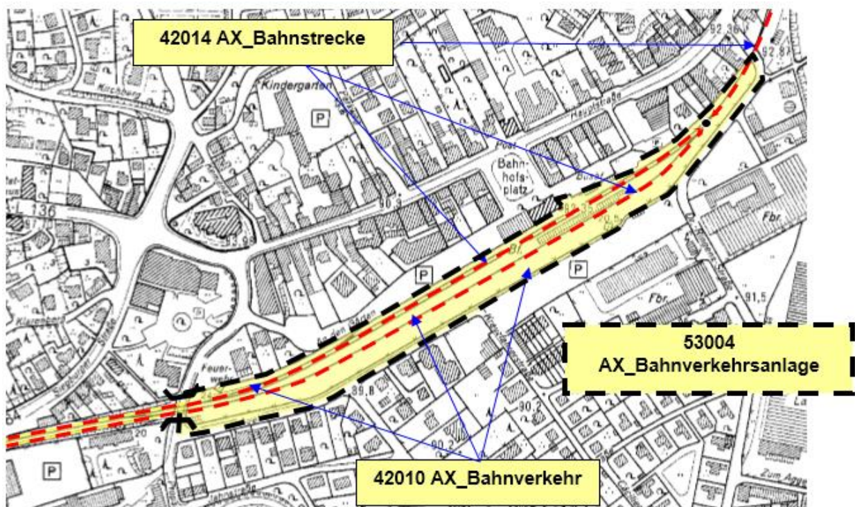
Abbildung 37: Modellierung mehrerer Bahnstrecken
