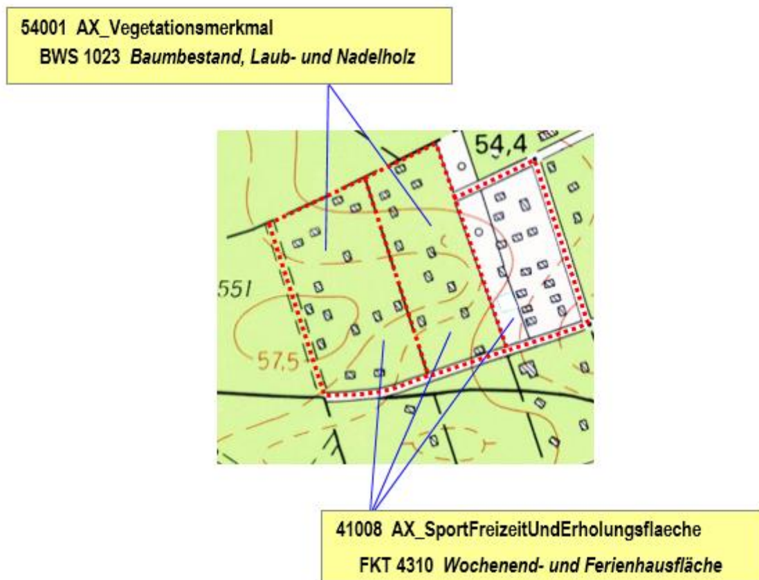
Abbildung 29: Beispiel für die Überlagerung einer Siedlungsfläche mit Vegetation
