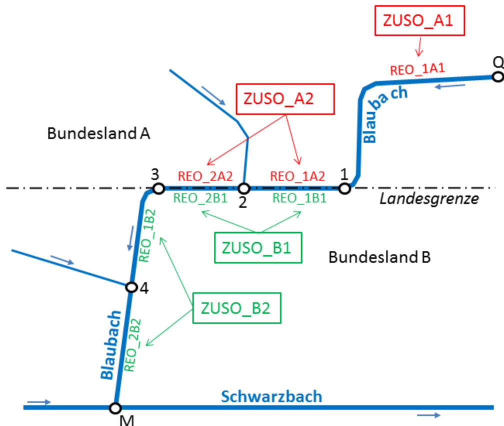
Abbildung 6: Beispiel für ZUSO- und REO-Bildungen an Landesgrenzen
