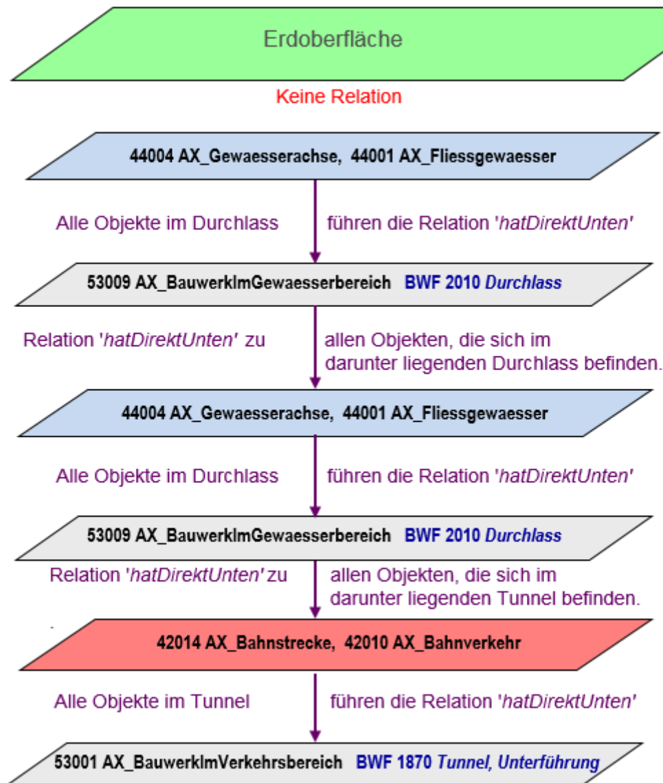
Abbildung 16: Vertikale Abbildung der Landschaft unter der Erdoberfläche
