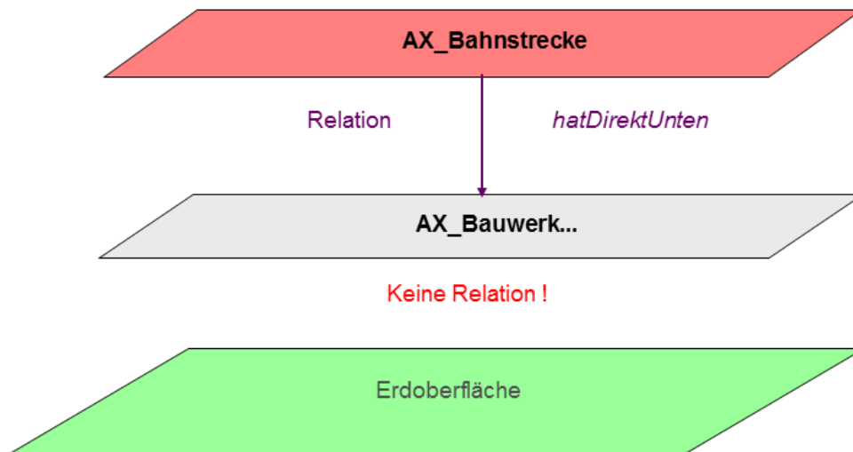
Abbildung 10: Vertikale Abbildung der Landschaft über der Erdoberfläche
