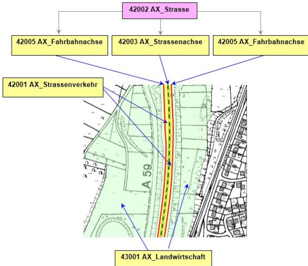
Abbildung 33: Modellierung einer Straße mit physisch getrennten Fahrbahnen
