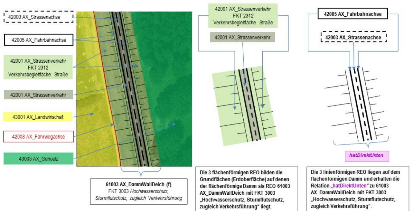
Abbildung 61: Modellierung eines flächenförmigen Damms mit Straßen- und Fahrbahnachsen
