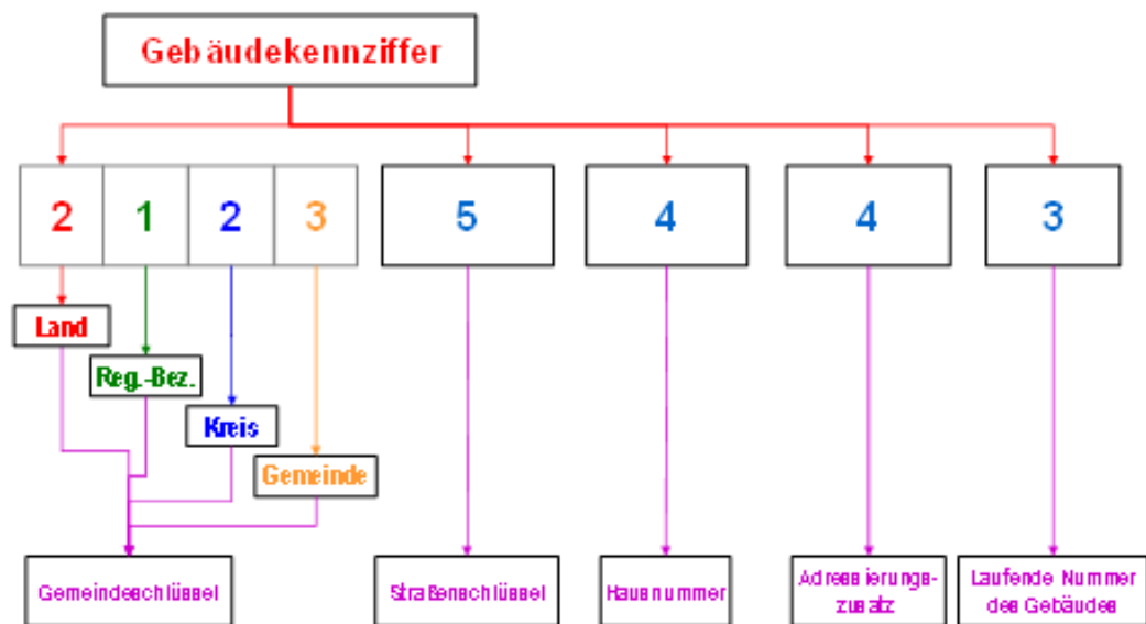
Abbildung 25: Aufbau des Gebäudekennzeichens
