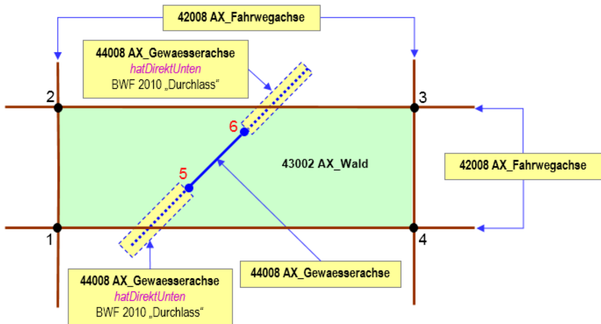
Abbildung 28: „Maschenbildner“ ohne Anbindung
