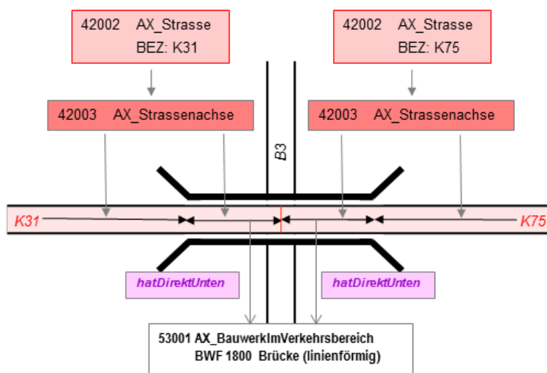
Abbildung 42: Modellierung einer linienförmigen Brücke
