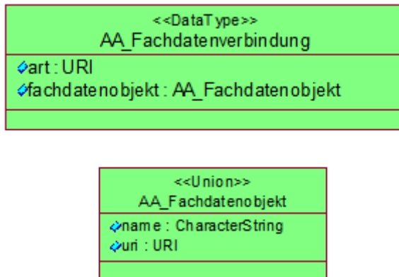
Abbildung 2: Modellierung der Fachdatenverbindung in UML
