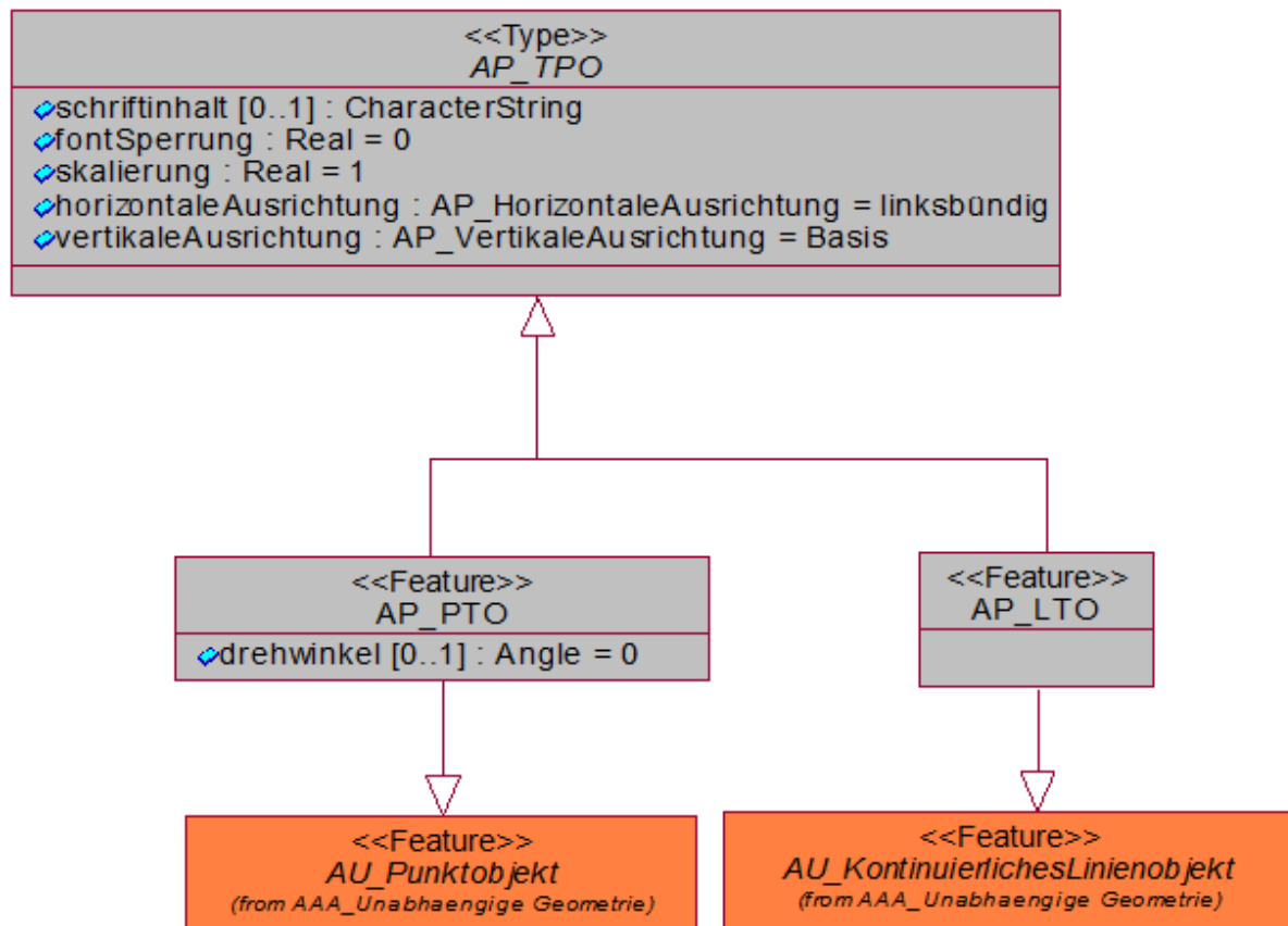
Abbildung 22: Auszug aus Basisschema, AP_TPO
