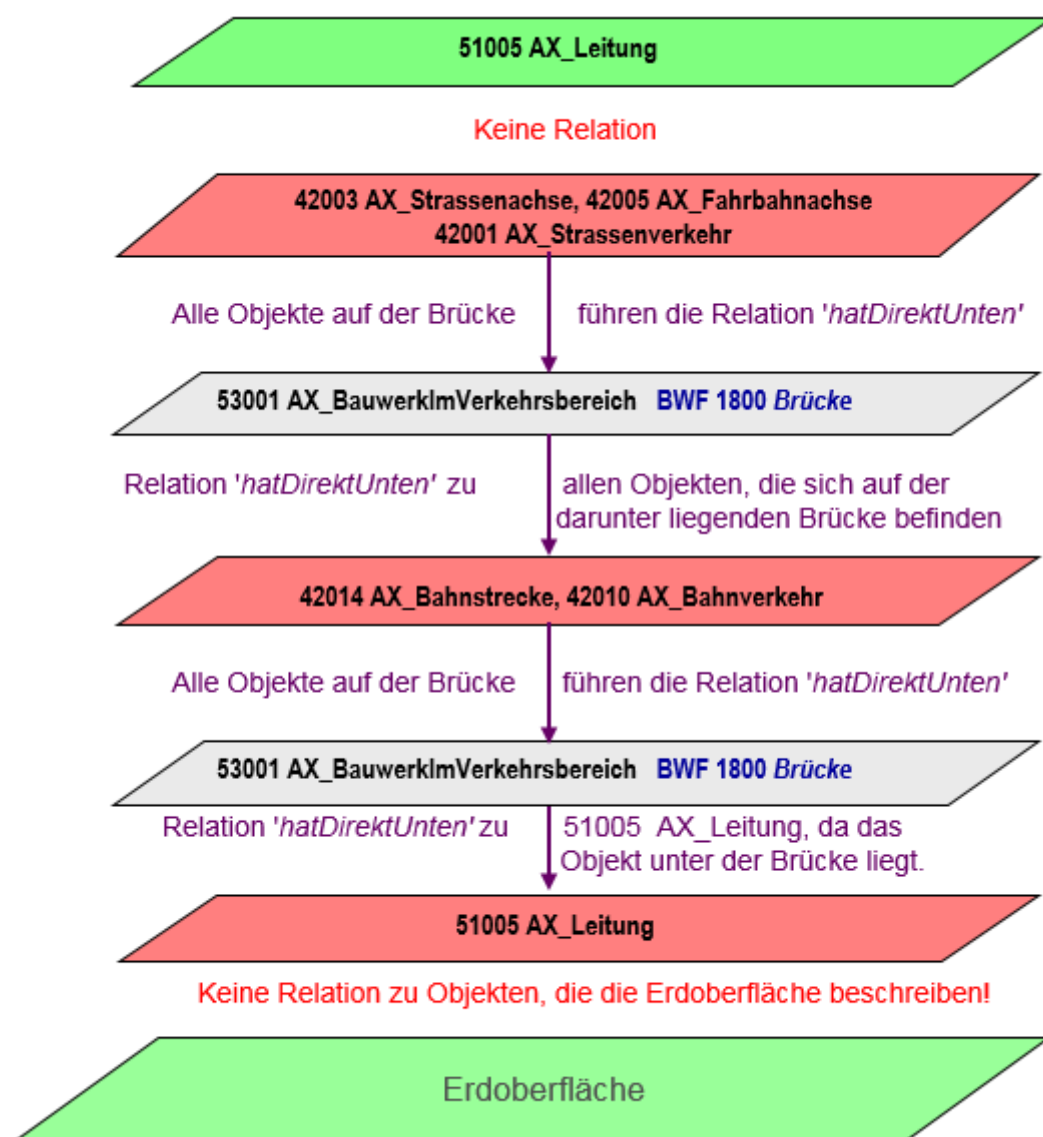
Abbildung 14: Vertikale Abbildung der Landschaft über der Erdoberfläche
