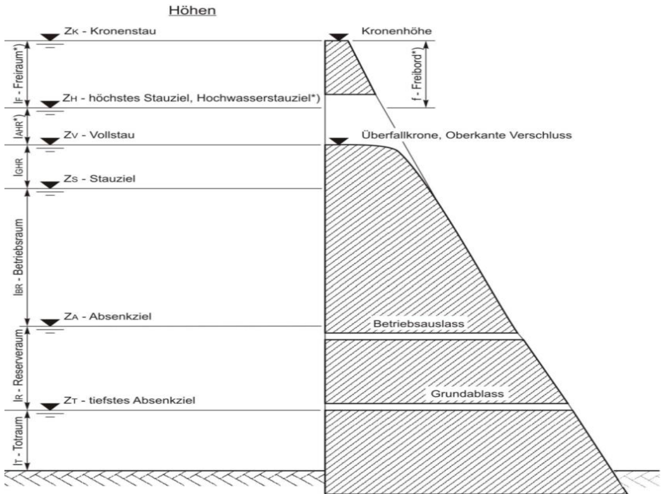
Abbildung 57: Schematische Darstellung der Stau- und Absenkeziele bei einem Stausee
