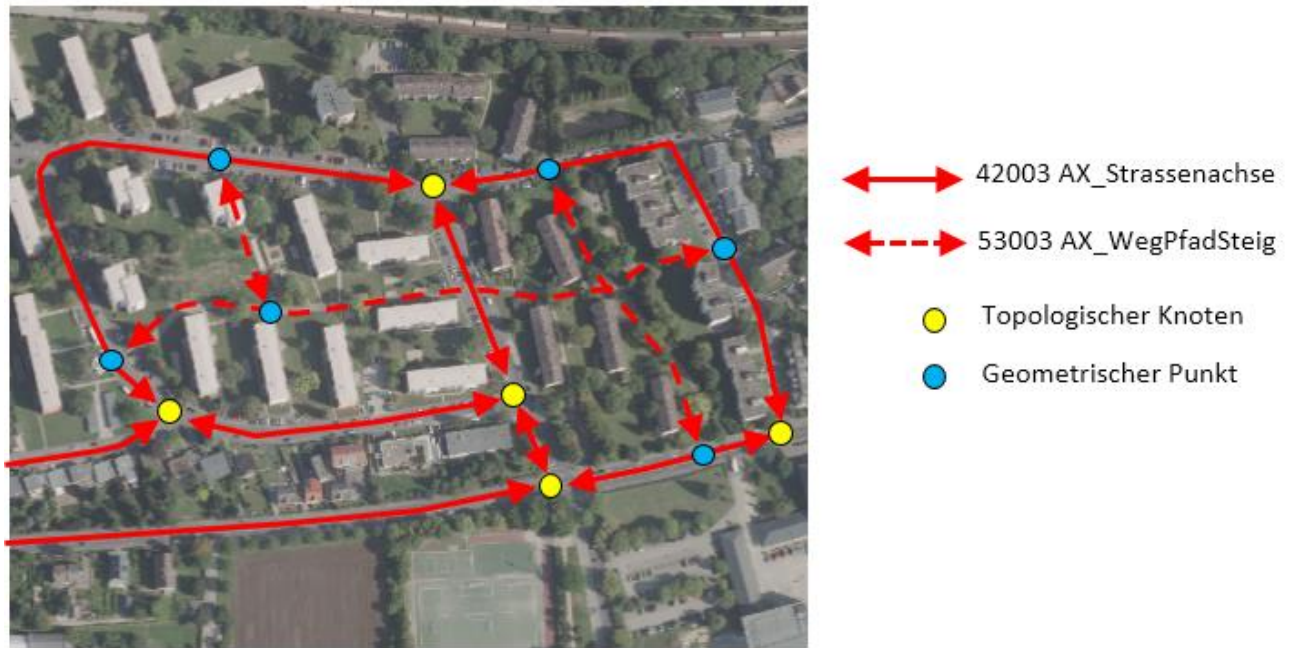
Abbildung 50: Modellierung von „Weg, Pfad, Steig“ mit Straßenachse
