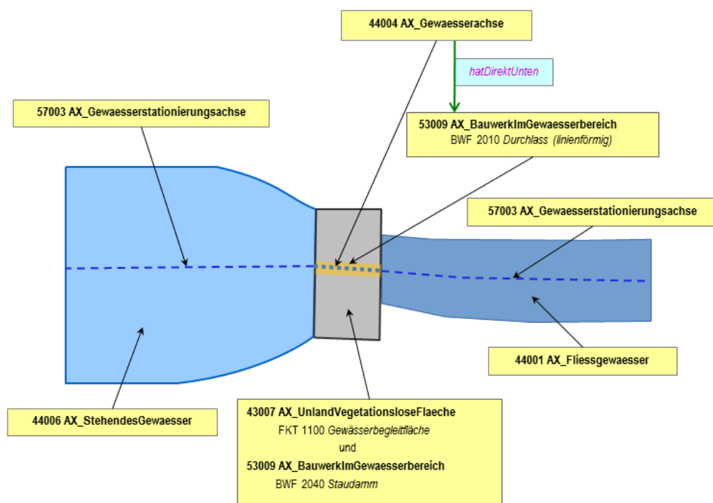
Abbildung 54: Modellierung von Wasserlauf unter Staudamm in linienförmigem Durchlass
