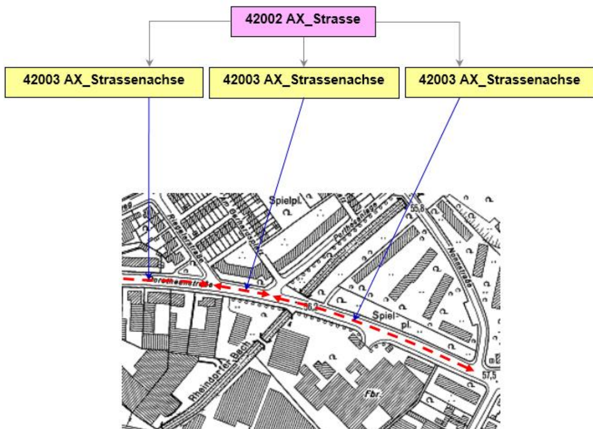
Abbildung 31: ZUSO AX_Strasse besteht aus 3 REO AX_Strassenachse
