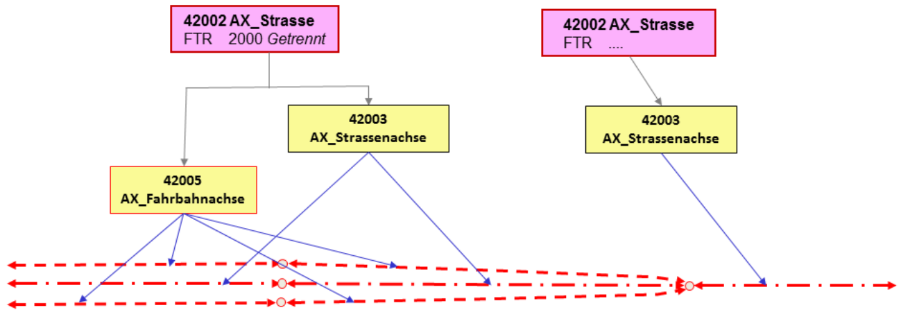
Abbildung 34: Modellierung eines „Übergangs“ physische Trennung in nicht-physische Trennung
