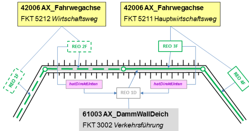
Abbildung 60: Modellierung eines linienförmigen Damms mit mehreren Fahrwegachsen
